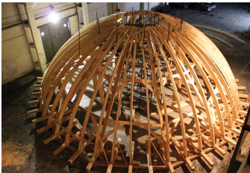
Obnova krovové konstrukce v kostele sv. Anny v Nových Dvorech
