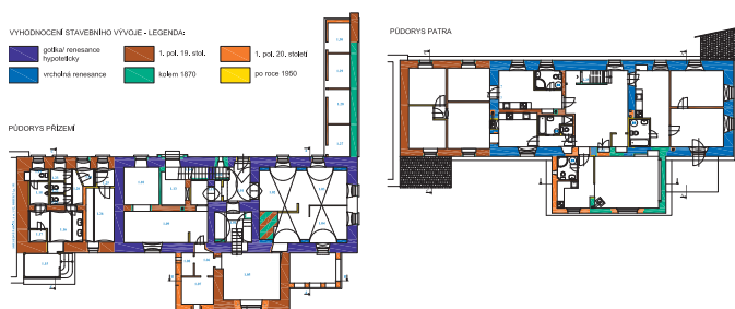
Olbramovice (okr. Benešov), dům čp. 1 – půdorysné plány s vyhodnocením stáří konstrukcí zpracované pro návrh na prohlášení domu za kulturní památku. S použitím plánové dokumentace O. Podojila, DiS., zpracoval a vyhodnotil Ing. arch. J. Veselý, 2016.
