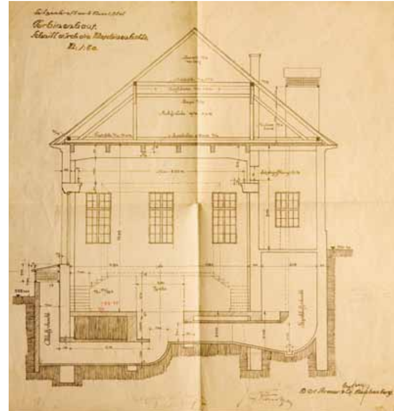
Příčný řez strojovnou s podzemní šachtou chlazení generátoru
