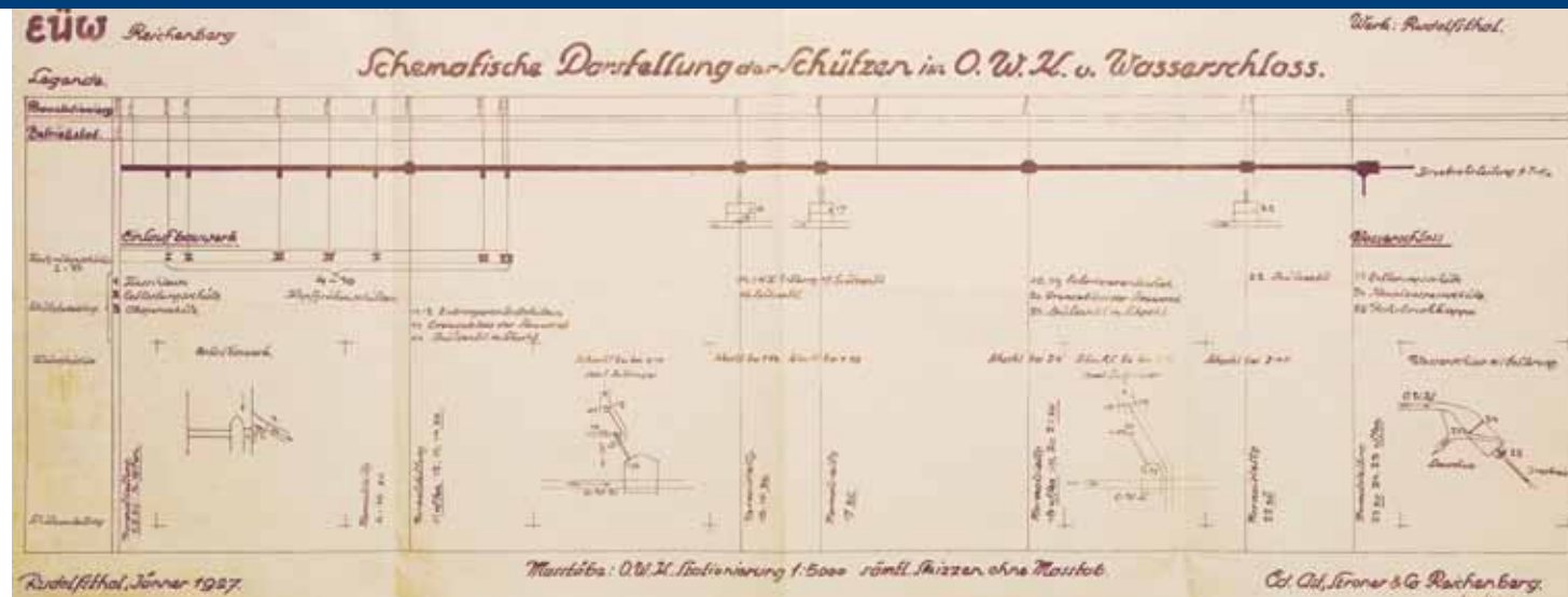
Schéma 3 251 m dlouhého úbočního přivaděče se situacemi objektů na trase
